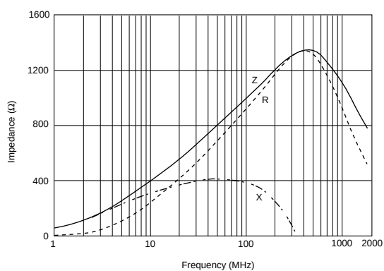
BLM18HK102SN1
