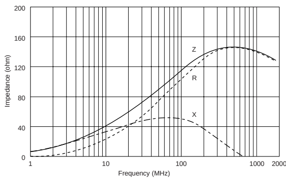
BLM18EG121SN1
