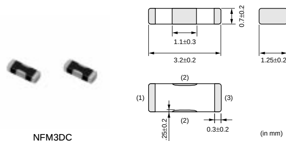
NFM3DC
