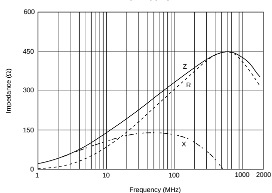
BLM18HK331SN1
