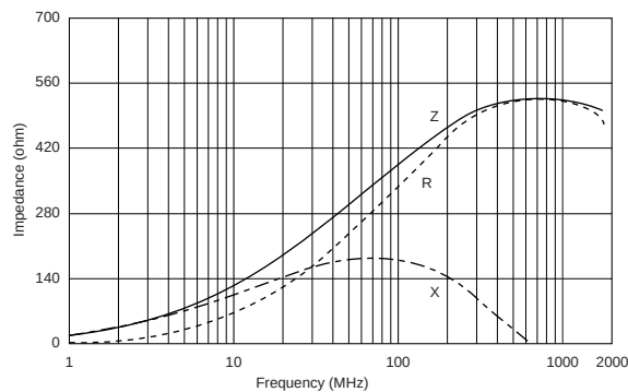
BLM18EG391TN1
