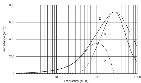
BLA2ABD471SN4
