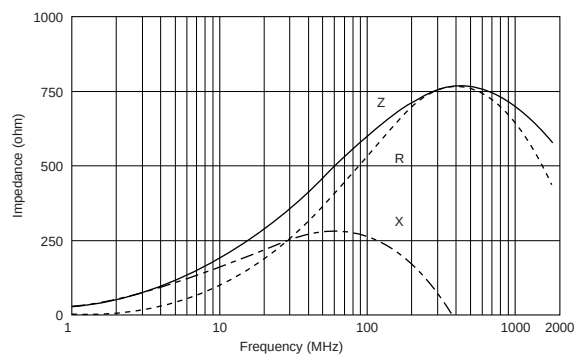
BLM18EG601SN1
