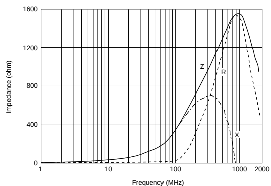
BLM18HB331SN1
